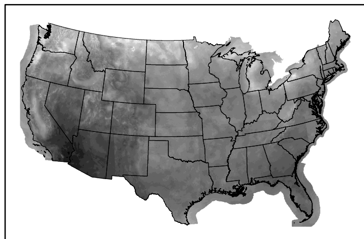
10hr Fuel Moisture mc10241201.bil
