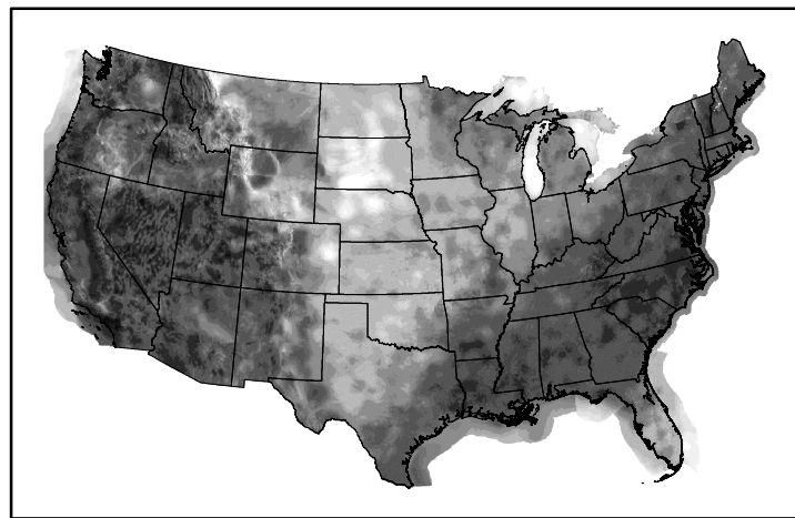
Wind Speed wspd20241026.bil
