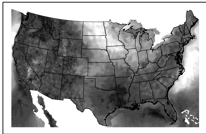
Wind Speed wspd20240606.bil
