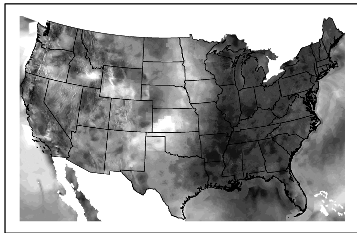
Wind Speed wspd20240602.bil
