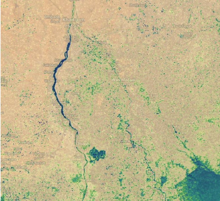
SSEBop VIIRS v6 Aug Dekad 1, 2023
