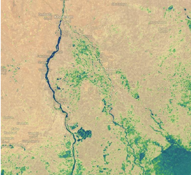
SSEBop VIIRS v6 Aug Dekad 2, 2023
