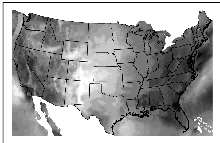
Wind Speed wspd20240506.bil
